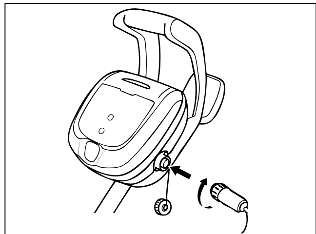
Figure 13. Brancher le câble électrique
